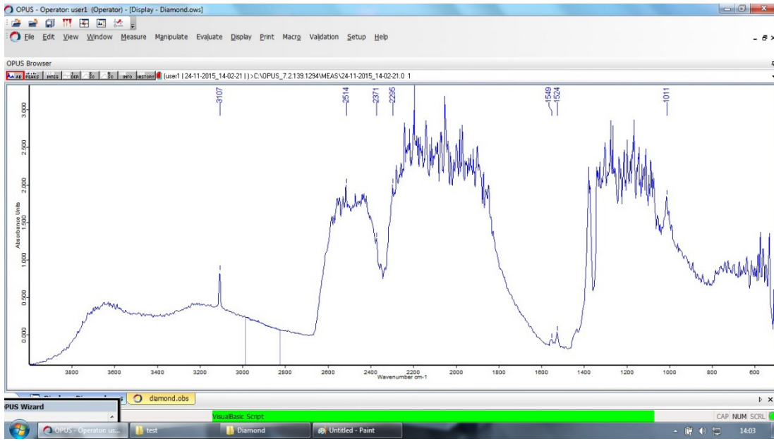
Grafik: 3 G1a sertifikalı Fancy Yellow 2,01 ct büyüklüğündeki taşın kızılötesi spektrumu
